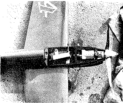
Fontana/Amodios installation med Super Tigre G15 diesel. Oljekylningens tid är tydligen förbi.
