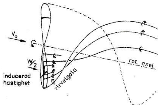
Fig. 3 Propellerns virvelsystem
