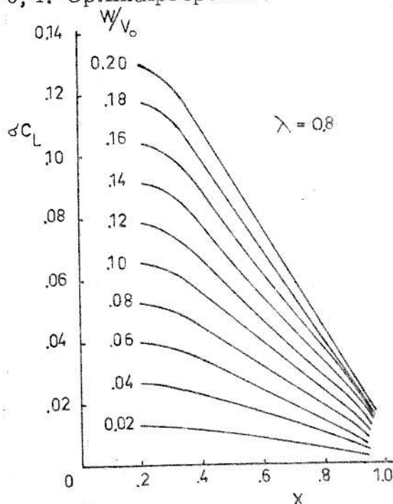
Fig. 9 \delta C_L som funktion av X och slipströmmens styrka för avanceringstalet \lambda = 0,8 . Optimalpropeller.
