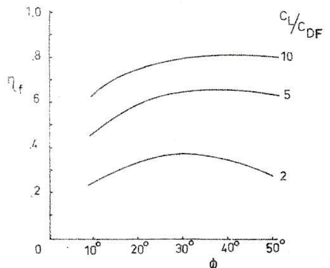
Fig. 5 Verkningsgrad för propellerbladelement
