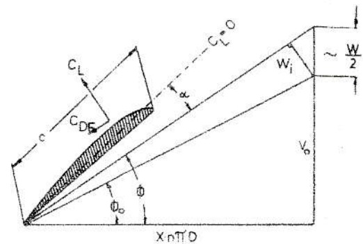
Fig. 4 Propellerbladelement
