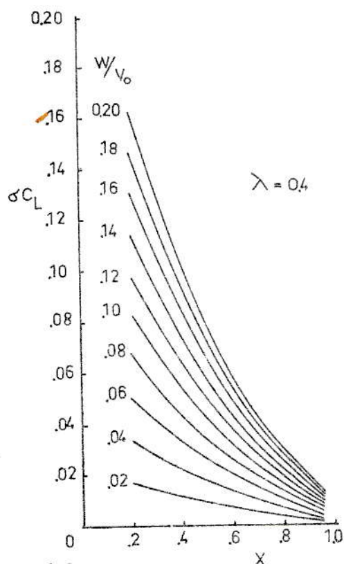
Fig. 8 \delta C_L som funktion av X och slipströmmens styrka för avanceringstalet \lambda = 0,4 . Optimalpropeller.
