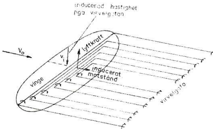
Fig. 2 Virvelsystem kring vinge
